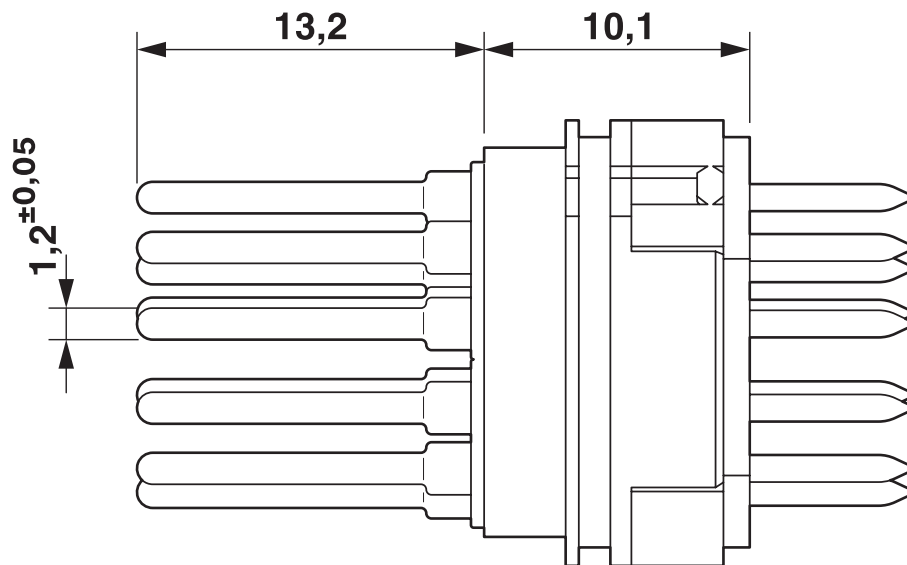
Dessin coté
