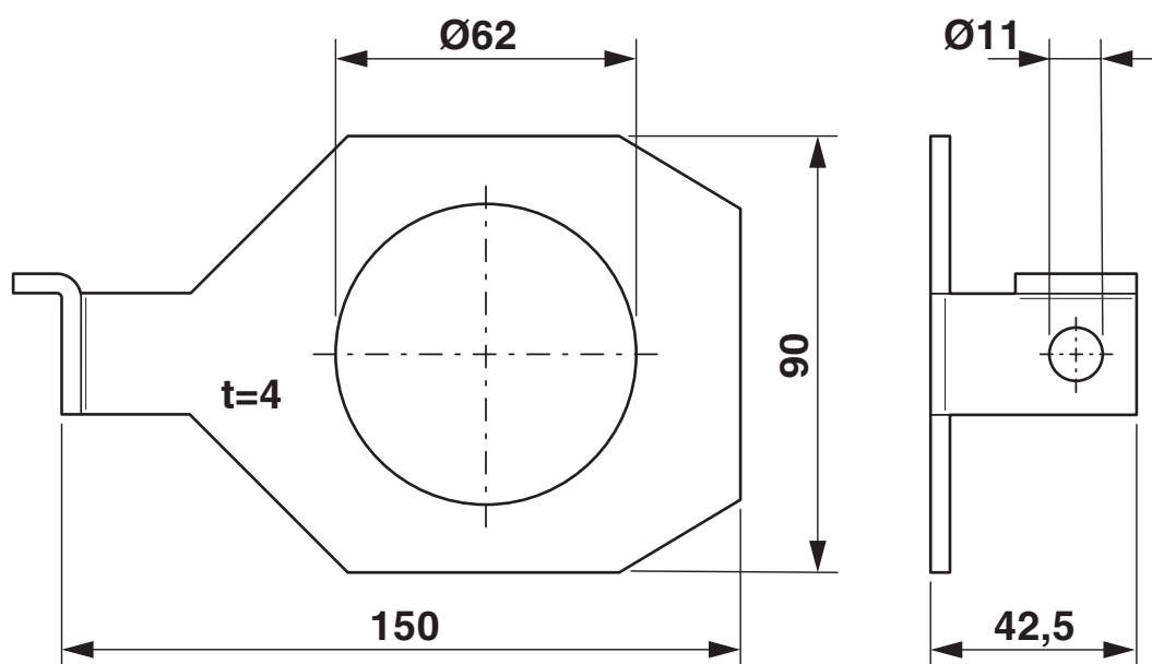
Dessin coté
