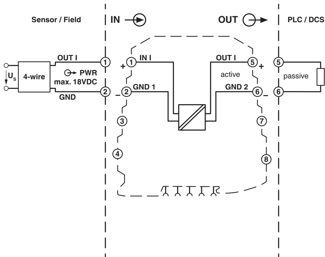
Schéma fonctionnel
