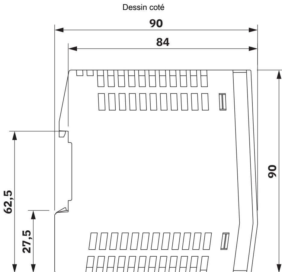
Encombrement de l'appareil (cotes en mm)
