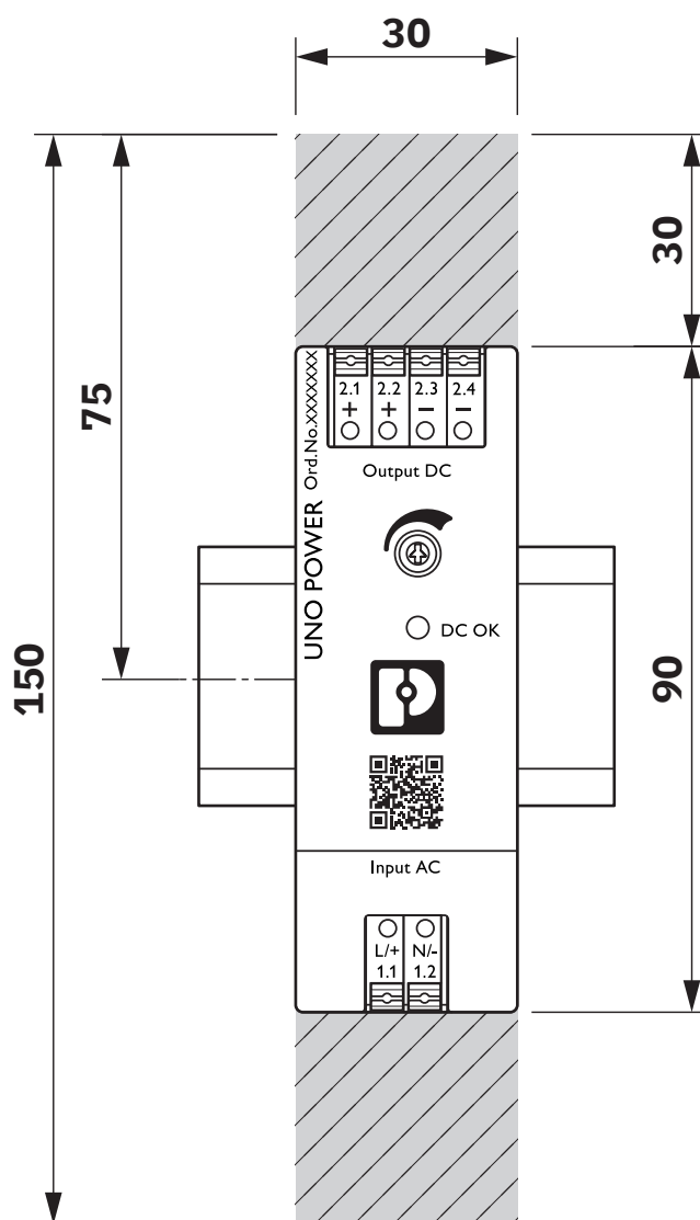
Dessin coté
