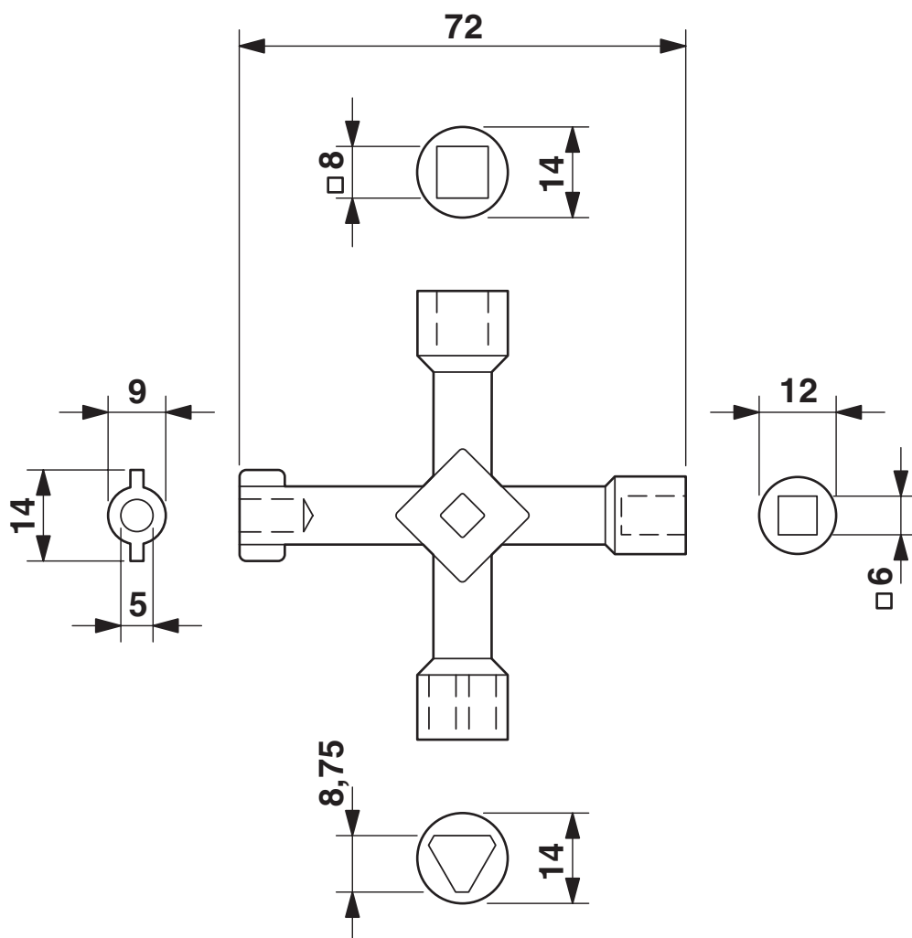
Maßzeichnung
