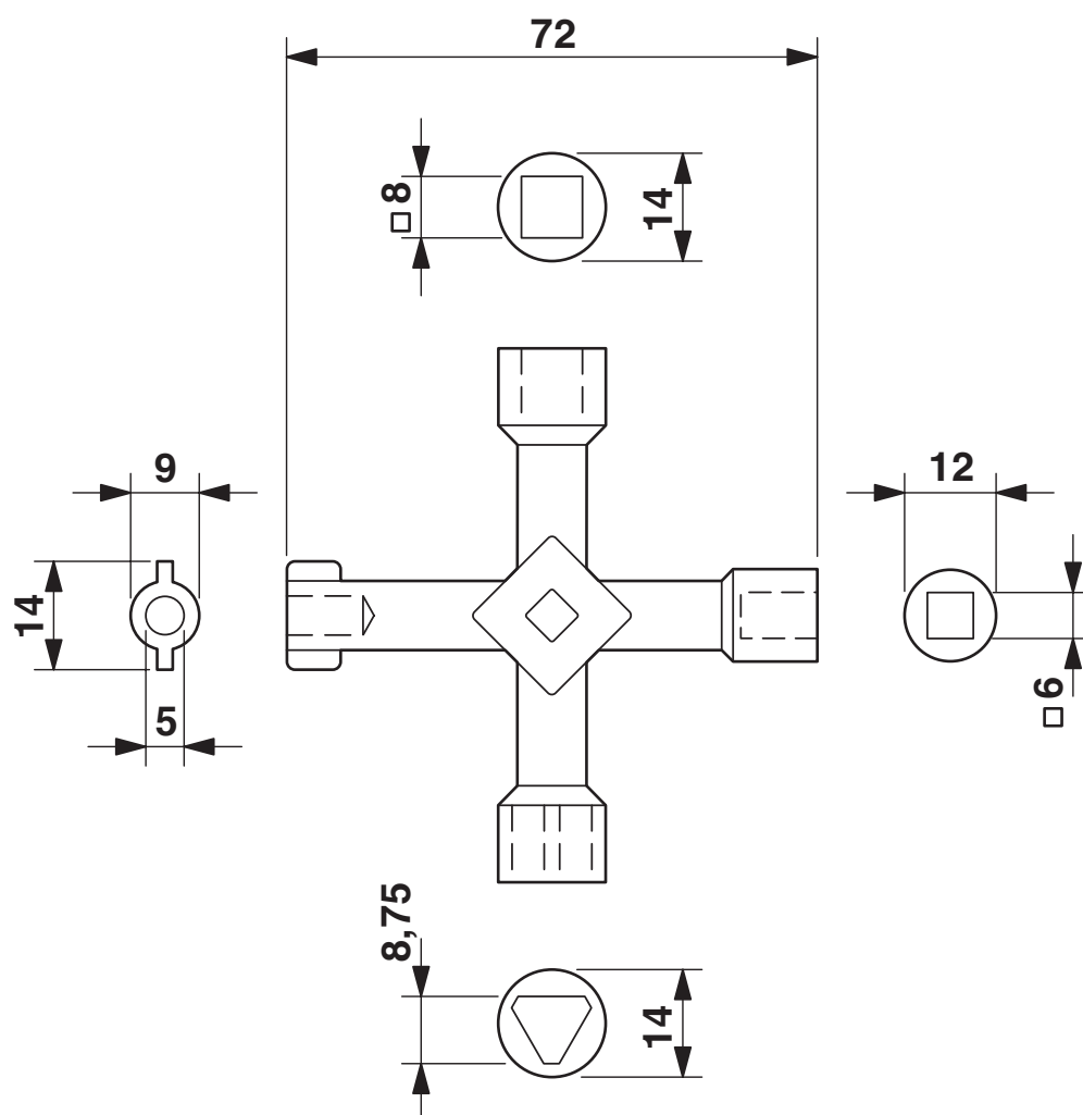
Dessin coté
