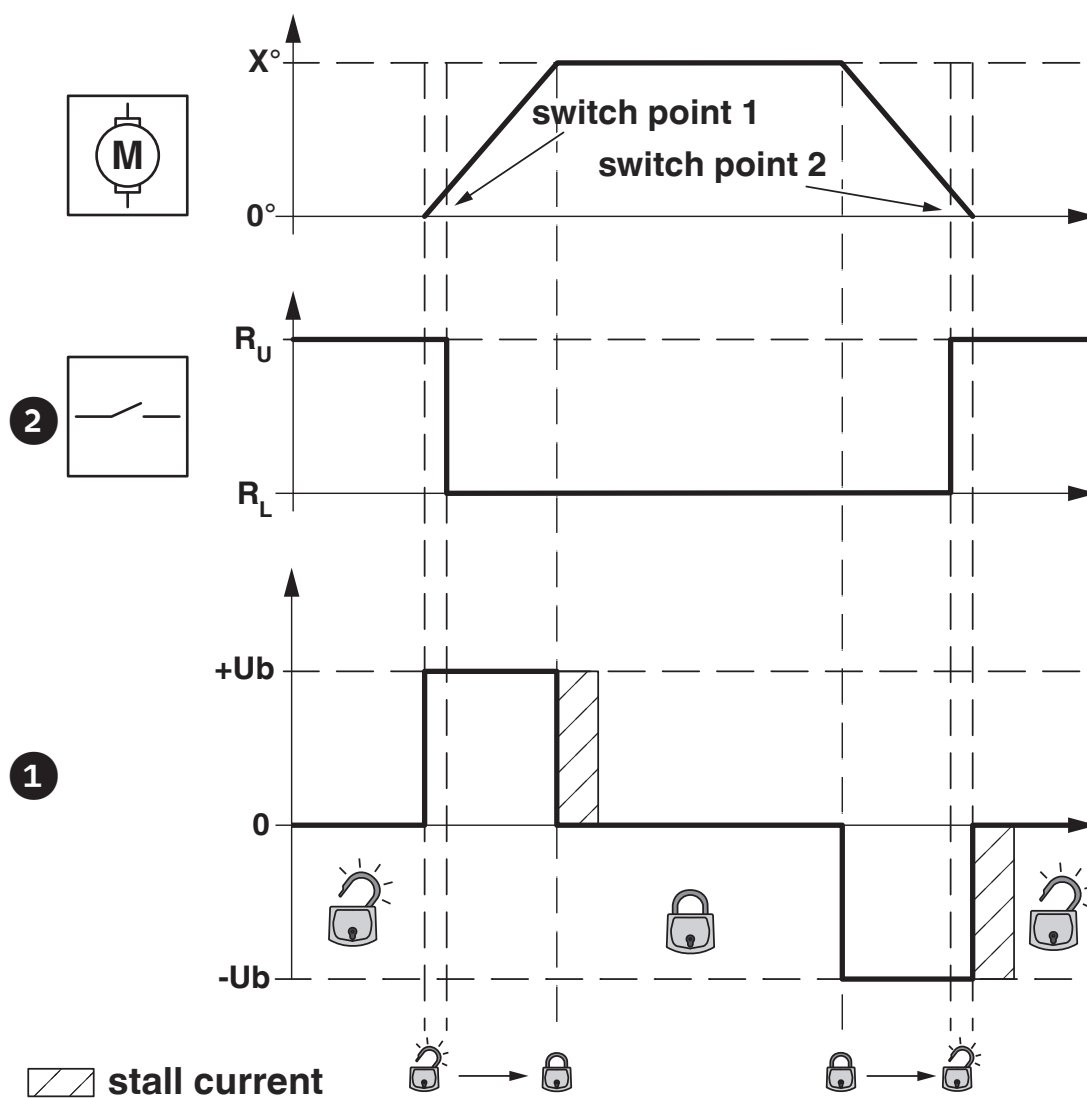
Schemazeichnung
