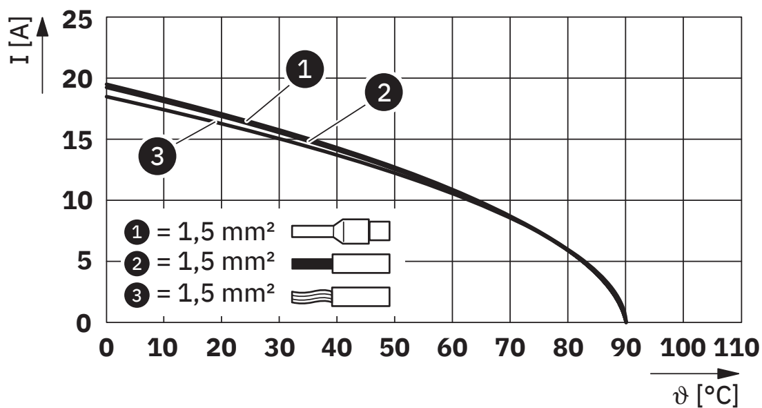
Diagrama derating para 1,5 mm²
