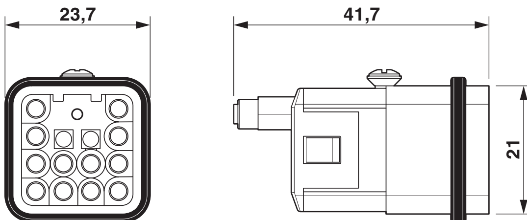
Maßzeichnung: HC-Q 12-I-CT-M
