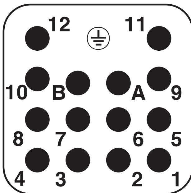
Polbild Anschlusseite. Position A und B für Kodierprofile
