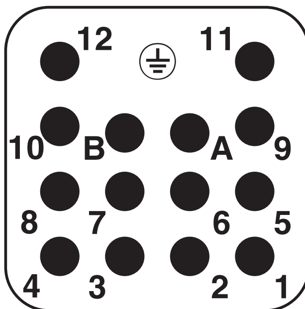
Dessin schématique
