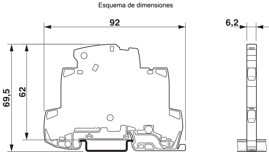
Plano esquemático
