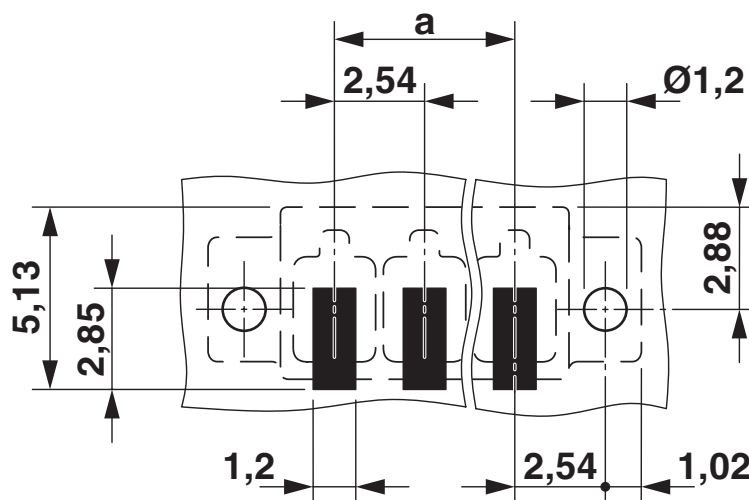
Bohrplan/Lötpadgeometrie
