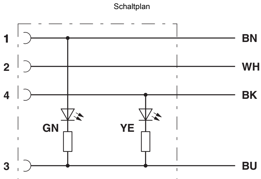
Kontaktbelegung der M8-Buchse mit LED
