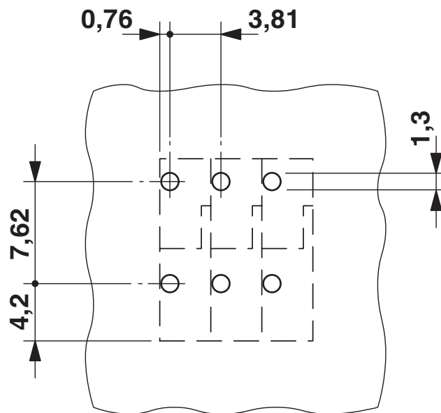
Bohrplan/Lötpadgeometrie
