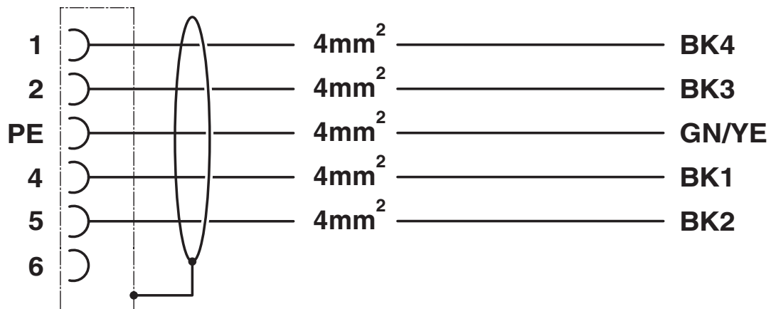
Diagrama eléctrico
