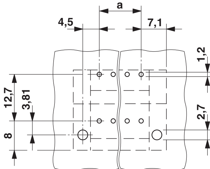
Bohrplan/Lötpadgeometrie
