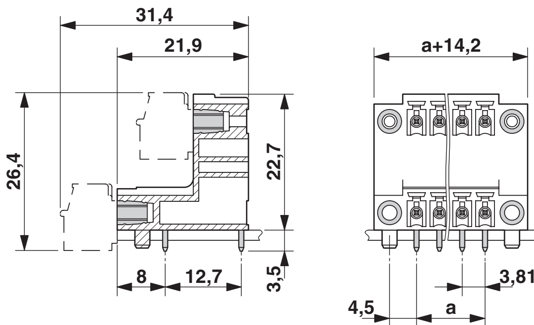
Dessin coté
