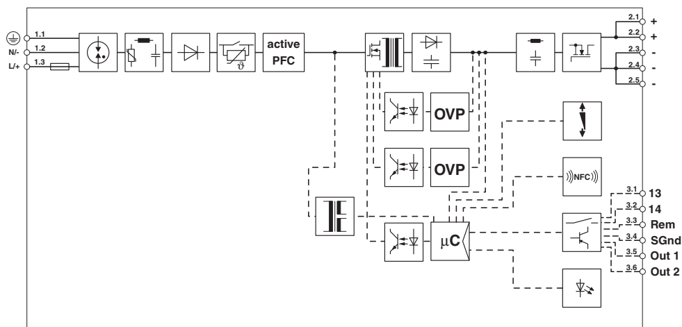
Blockschaltbild
