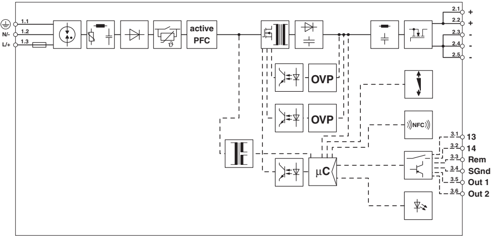
Schéma fonctionnel
