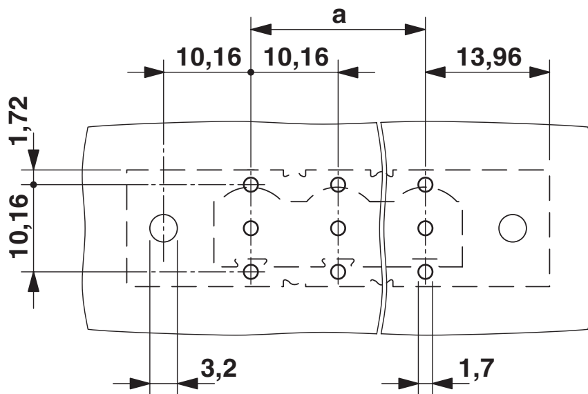
Bohrplan/Lötpadgeometrie
