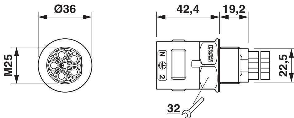
Dibujo acotado QPD W 4PE6,0 M25
