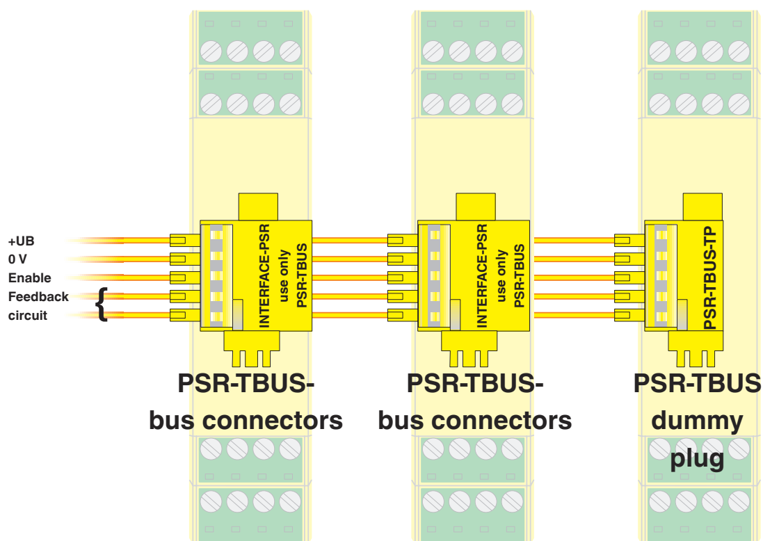
Anschlusszeichnung
