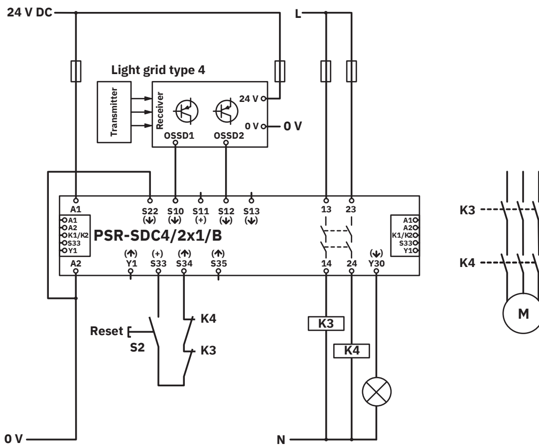
Schaltplan
