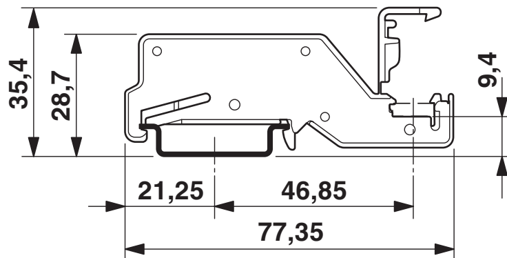
Dessin coté
