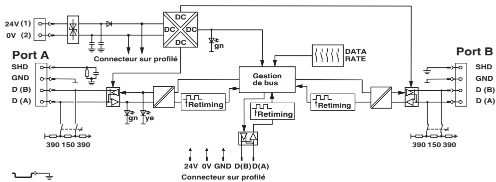
Schéma fonctionnel
