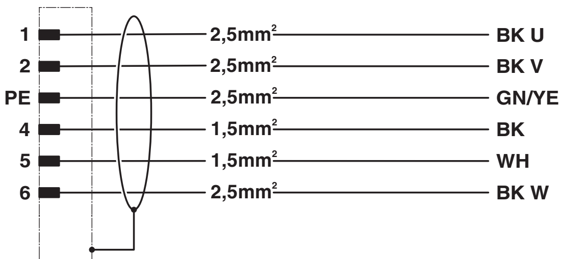
Schaltplan
