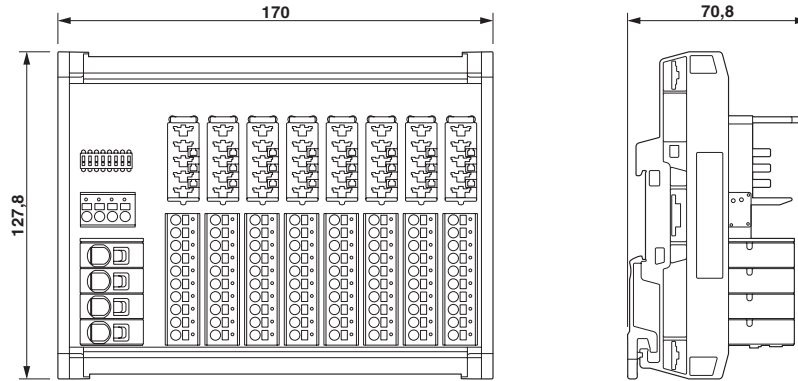
Maßzeichnung
