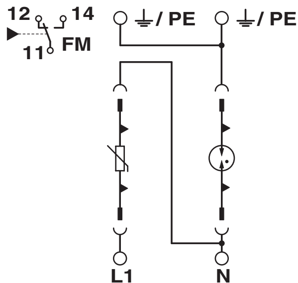
Schaltplan
