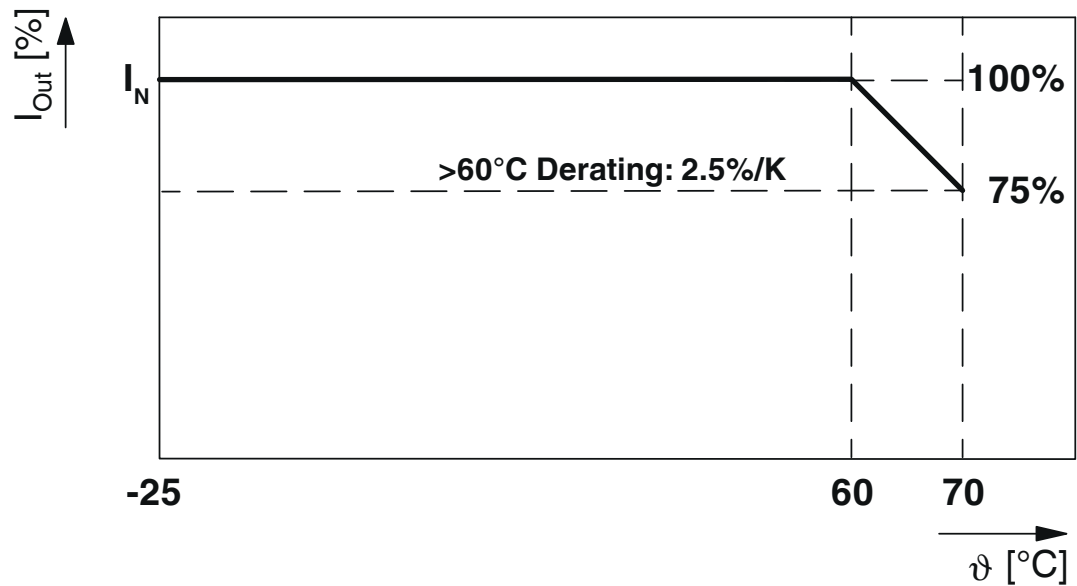
Ausgangsstrom/Umgebungstemperatur
