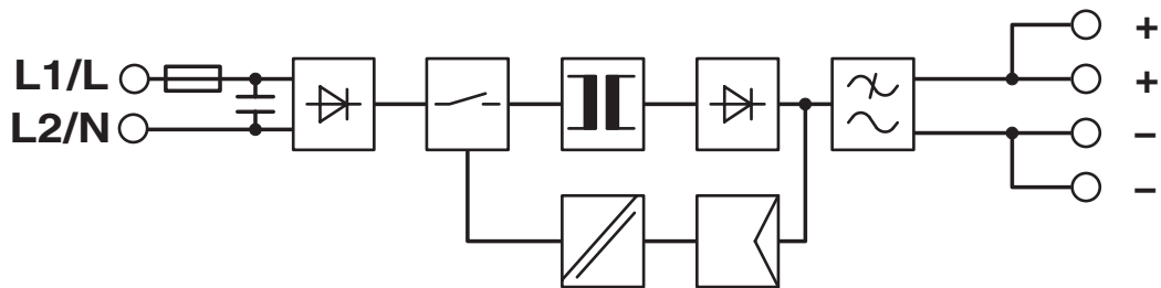
Blockschaltbild
