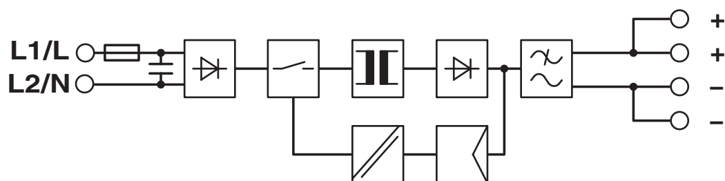
Esquema de conjunto
