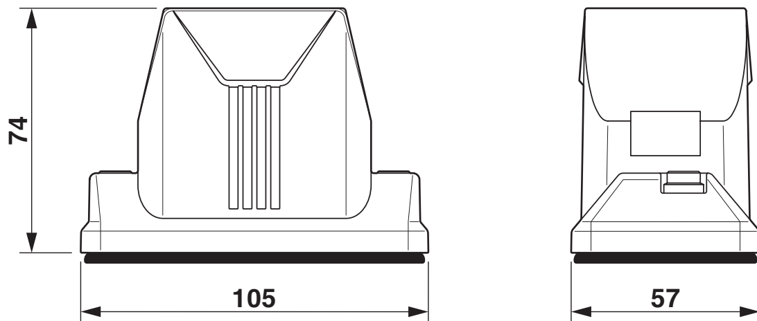
Maßzeichnung
