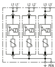
Schema di circuito basilare DG MP TNC 275 FM
