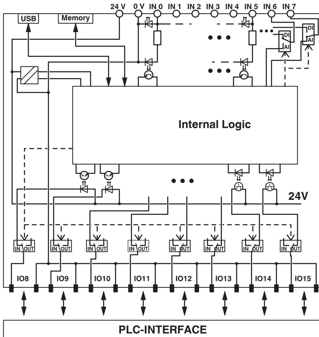
Schaltplan
