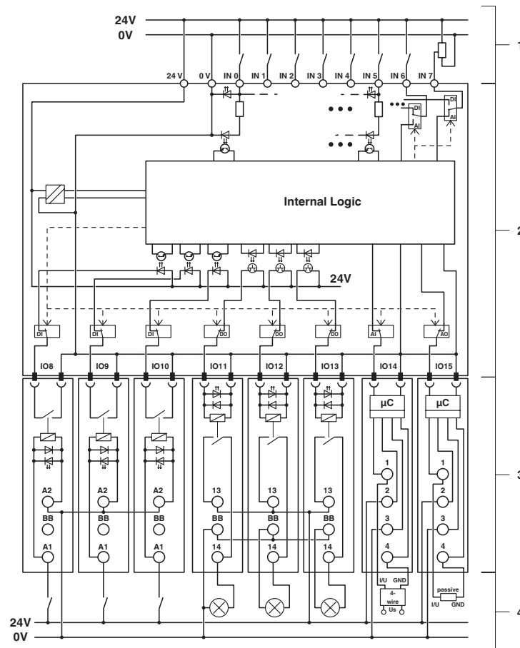
Diagrama eléctrico
