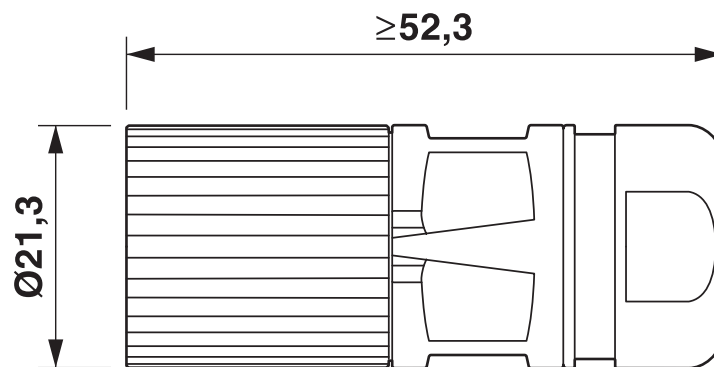
Dessin coté
