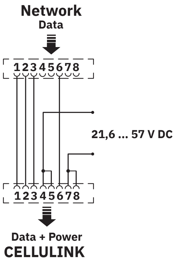
Anschlusszeichnung
