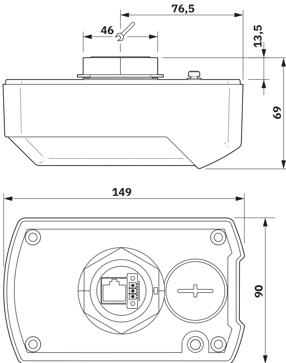
Maßzeichnung
