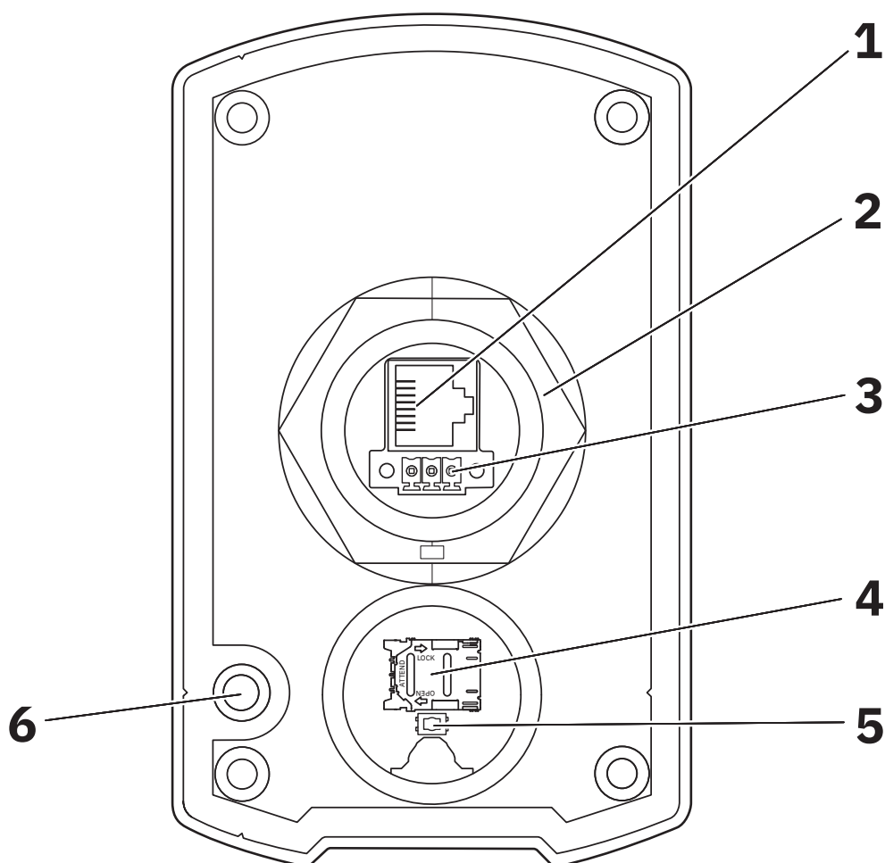
Plano esquemático
