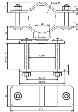
Maßbild BS D40.50 4K60.120 V2A
