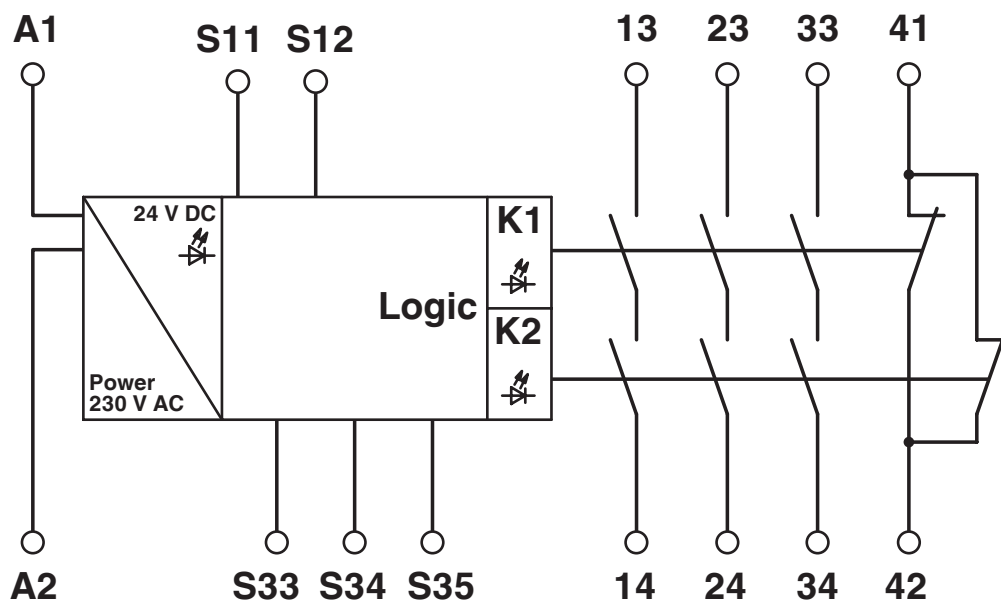
Diagrama eléctrico
