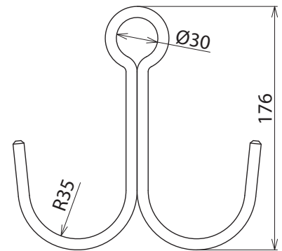
Maßbild EHH BEV OL
