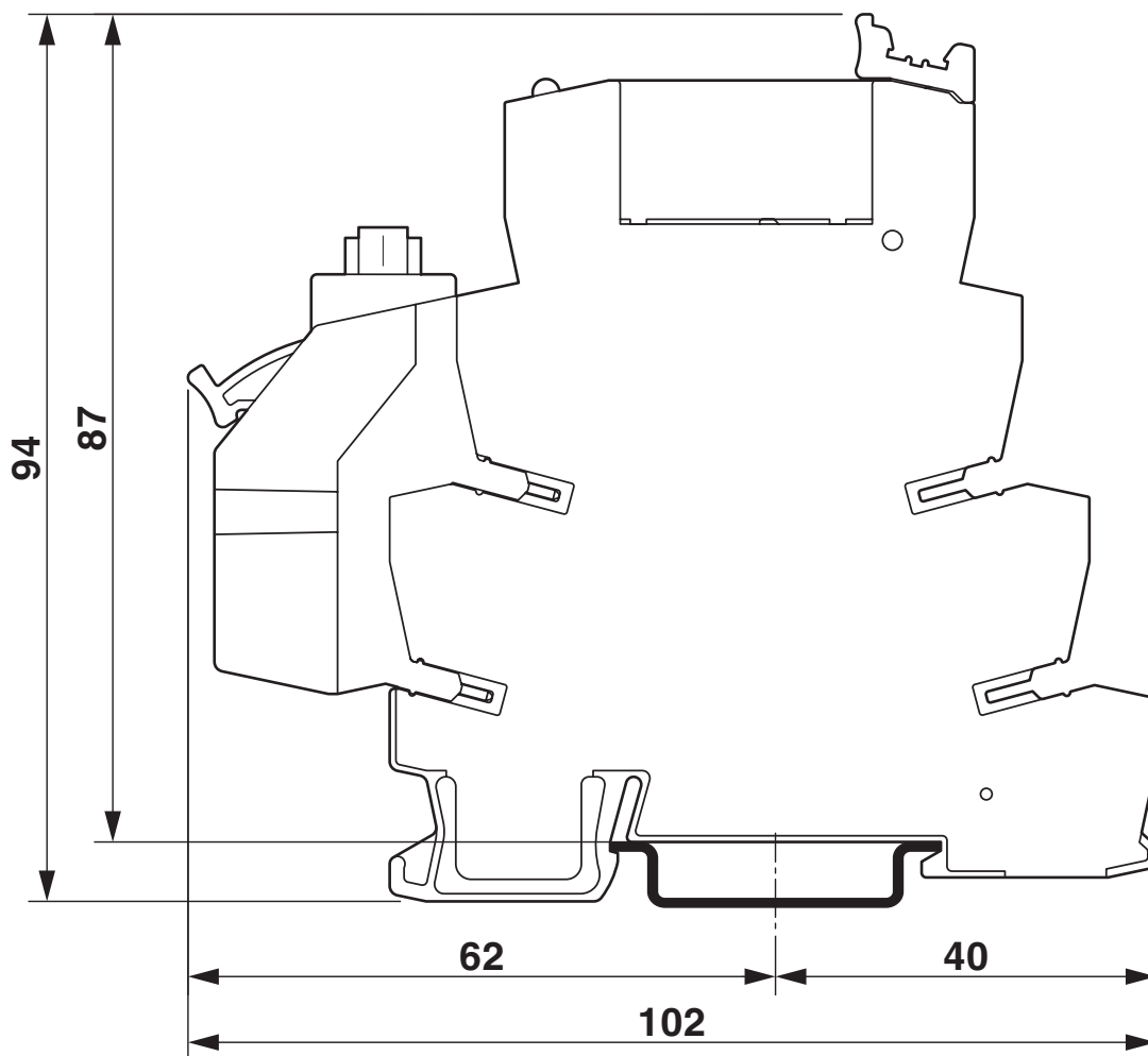
Maßzeichnung
