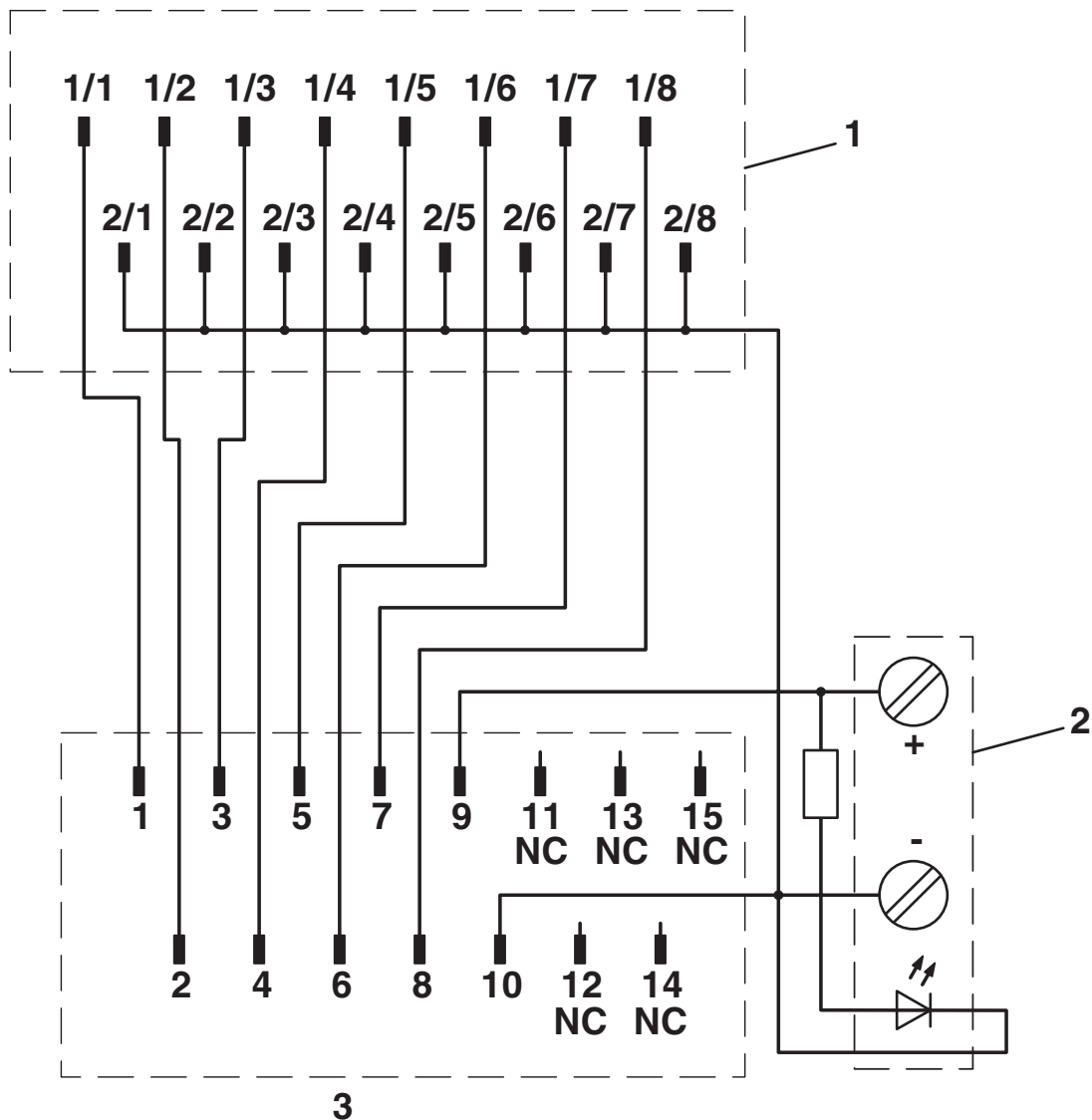
Diagrama eléctrico
