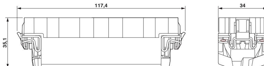
Dessin coté
