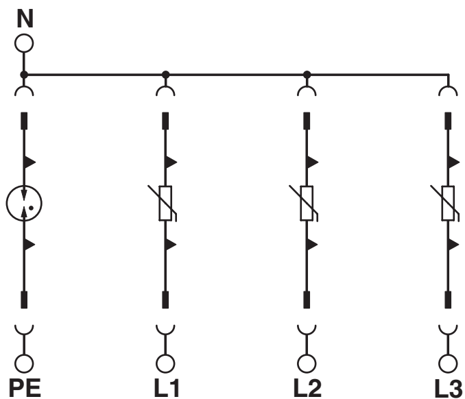
Diagrama eléctrico
