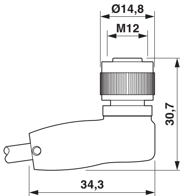
Dessin coté
