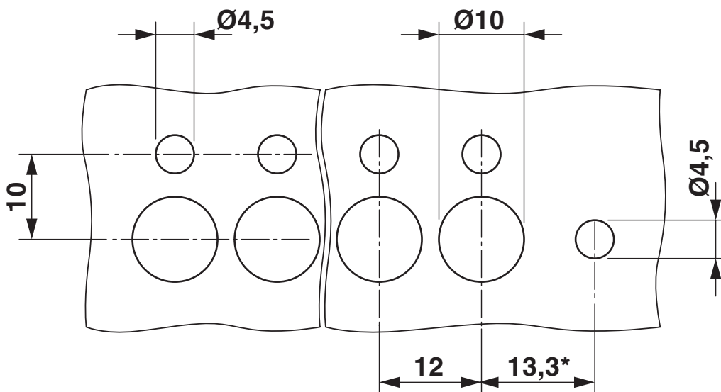
Maßzeichnung
