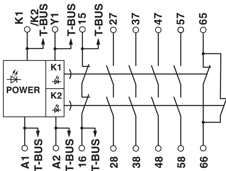
Diagrama eléctrico
