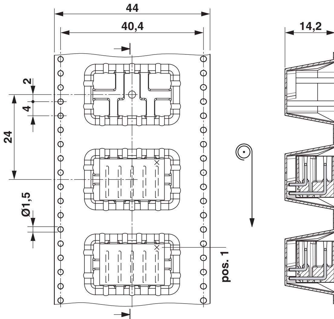
Maßzeichnung
