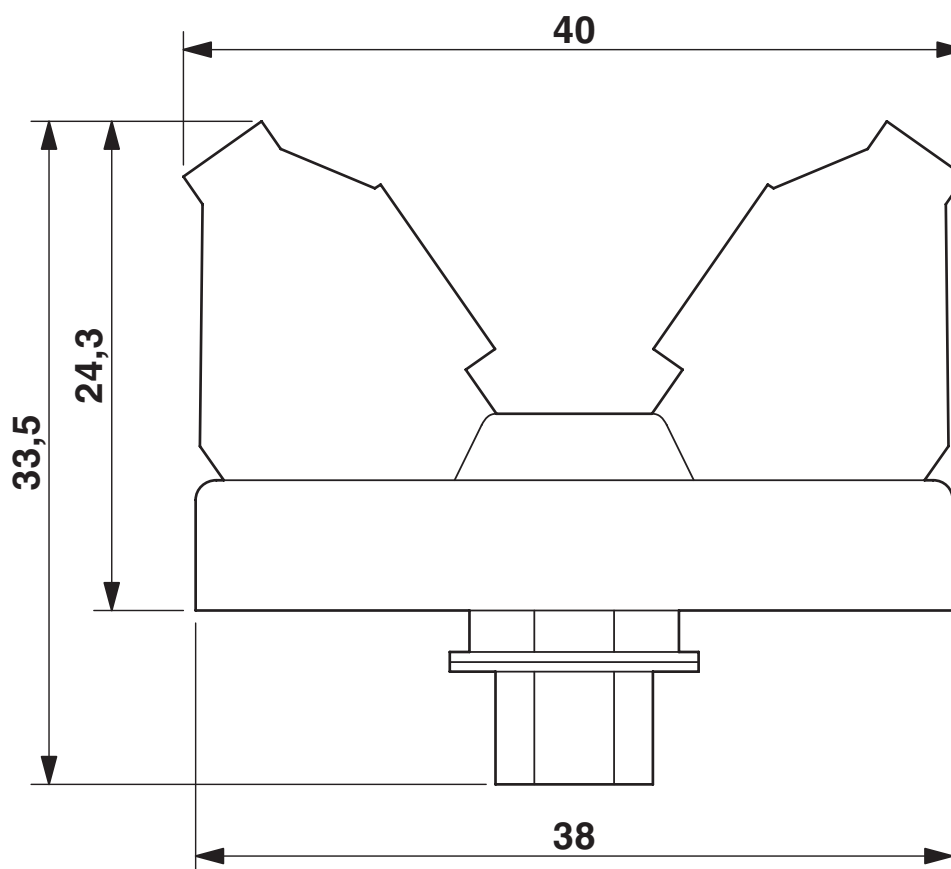
Dessin coté
