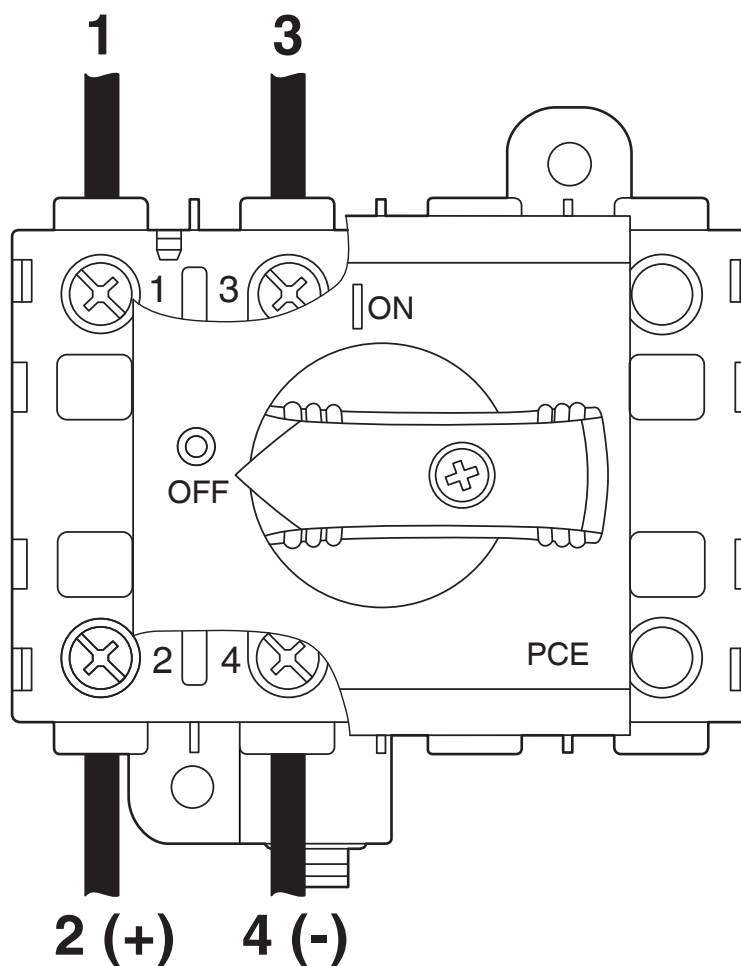
Anschlusszeichnung
